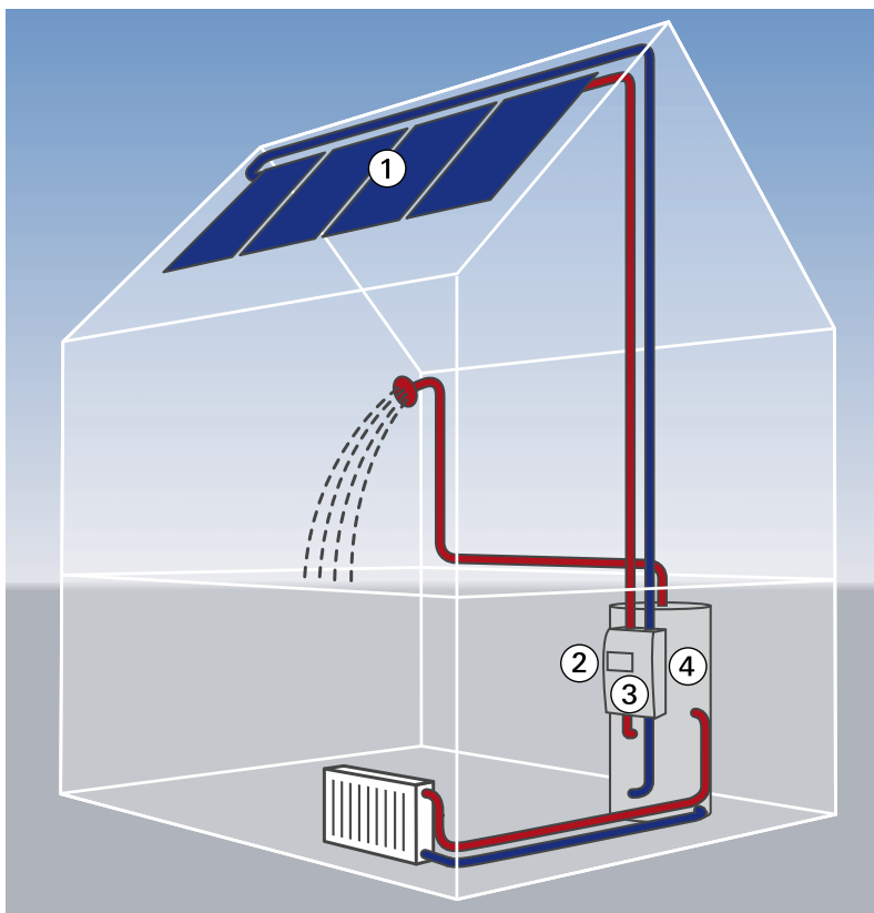
Schema Heizungsunterstützung
